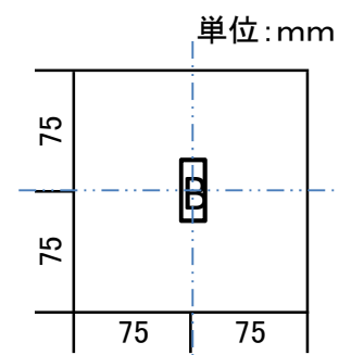
分電盤配置図
